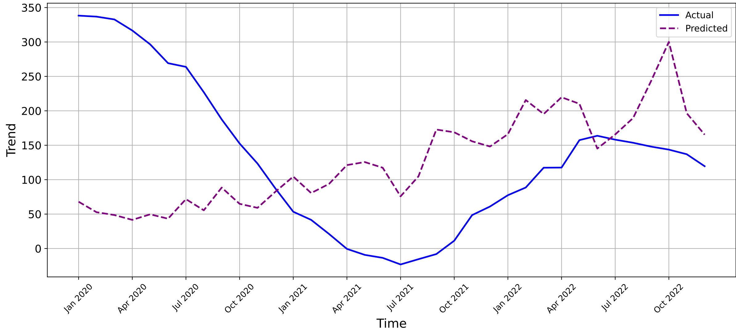
Trojan-ALL - Testing
